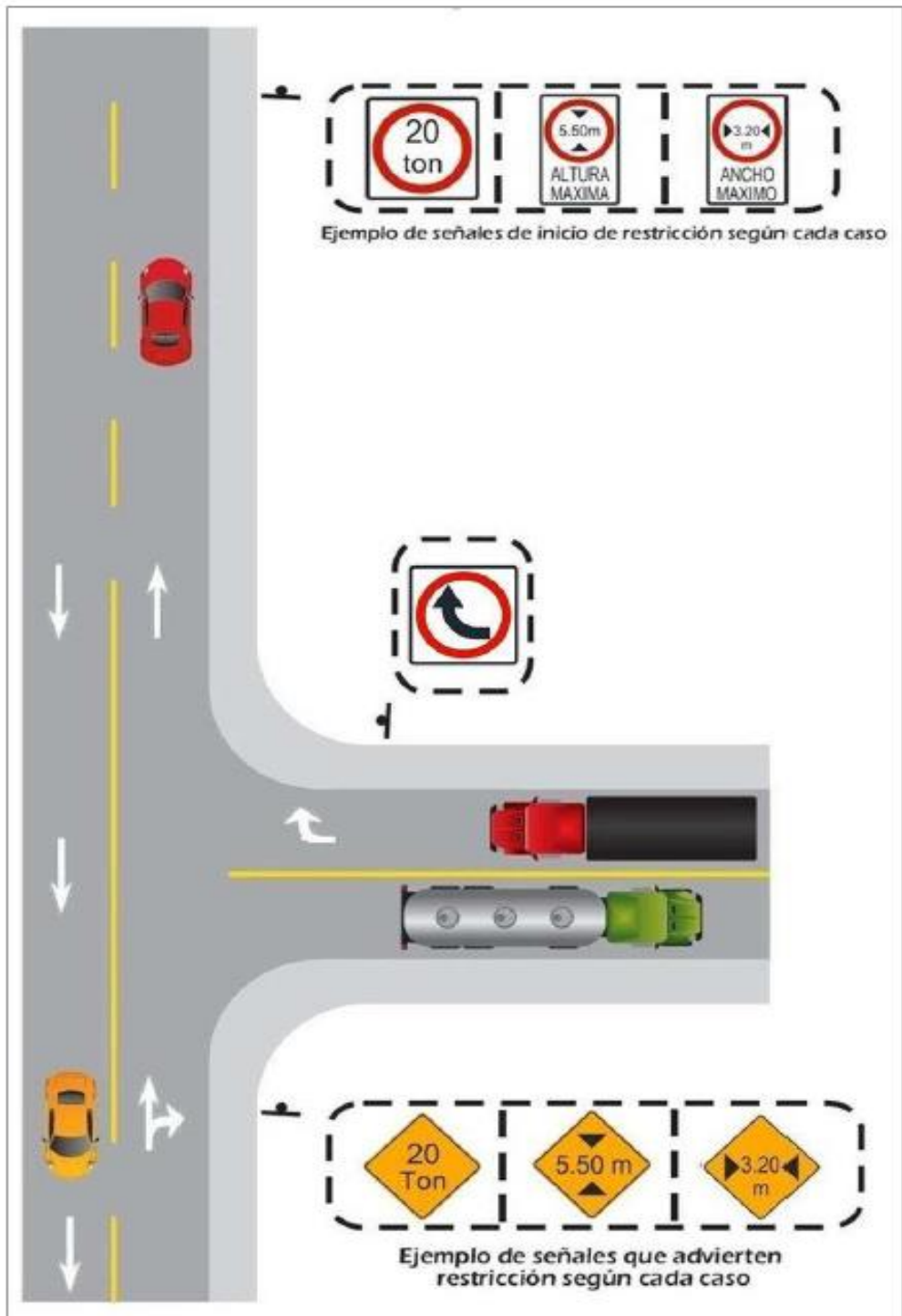
Imagen 14. Ejemplos de señales preventivas de restricción
