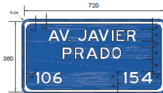
Imagen 35. Ejemplo de señales de identificación en zonas urbanas.
