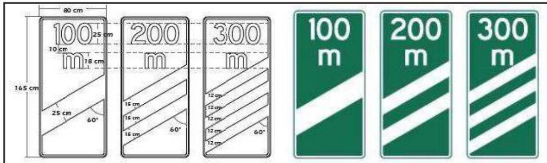
Imagen 29. Balizas de Acercamiento
