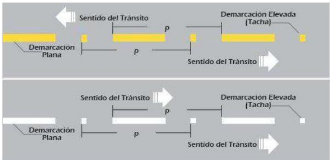
Imagen 69. Patrón de líneas Segmentadas "p"
