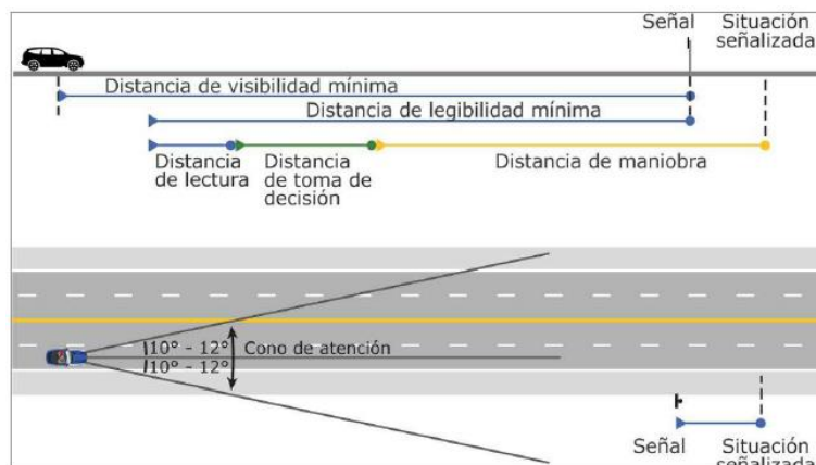
Imagen 5. Ubicación Longitudinal y Distancias de Lectura
