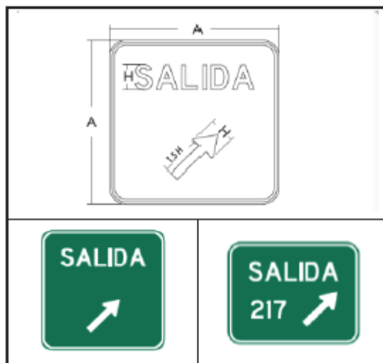
Imagen 30. Ejemplo de señales salida inmediata
