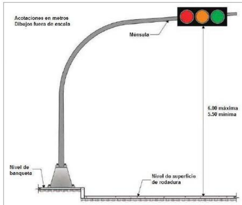
Imagen 71. soporte de semáforo tipo ménsula
