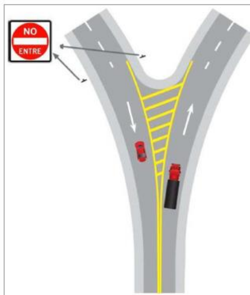
Imagen 40. Aplicación de señal NO ENTRE en intersecciones en "Y".
