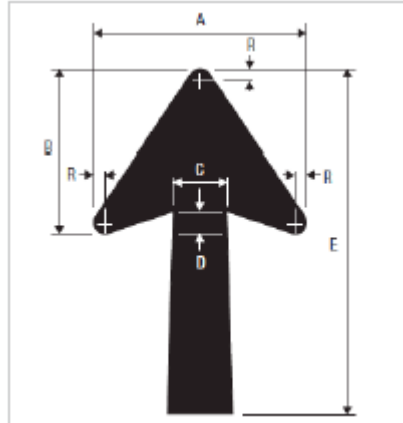
Imagen 23. Dimensiones de Flecha de destino
