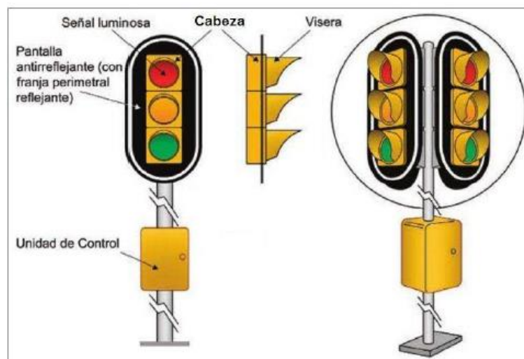
Imagen 72. configuración de cabeza de semáforos
