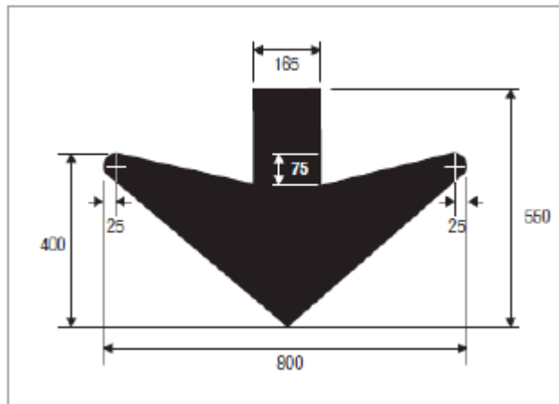
Imagen 25. Dimensiones de flecha descendente en señales aéreas.
