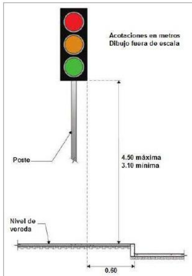
Imagen 70. soporte de semáforo tipo poste
