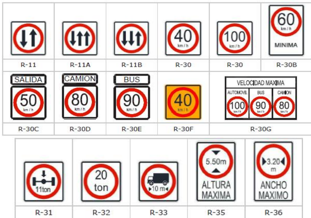
Imagen 11. Señales de restricción
